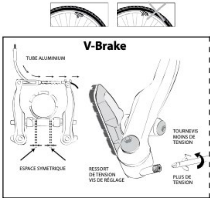
Le système de frein
